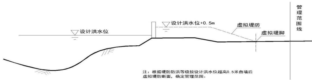
堤防直接为防洪墙段
