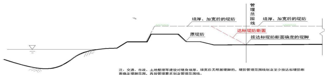
堤身培厚、加宽后无明显堤脚
